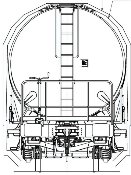
Gabarit d'encombrement
