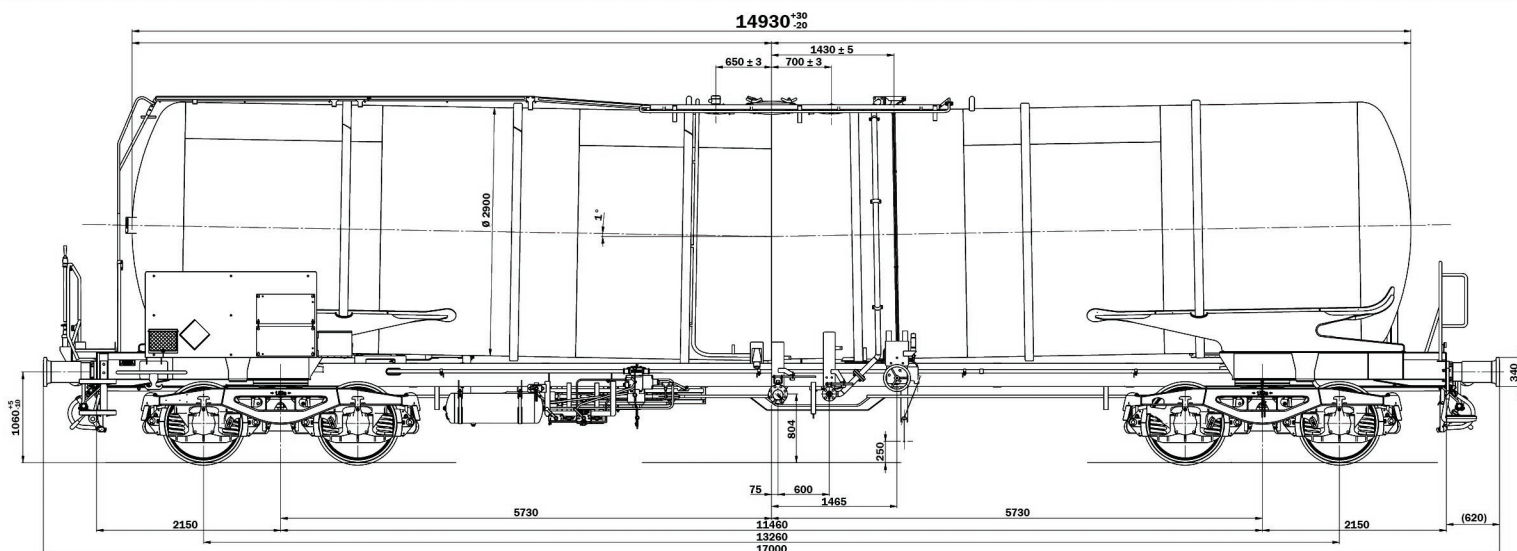
Gabarit de référence selon TSI Annexe C, figure C15
