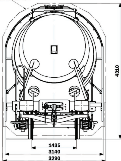
Gabarit 505-1
