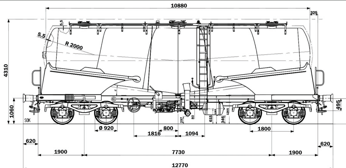
Gabarit 505-1
