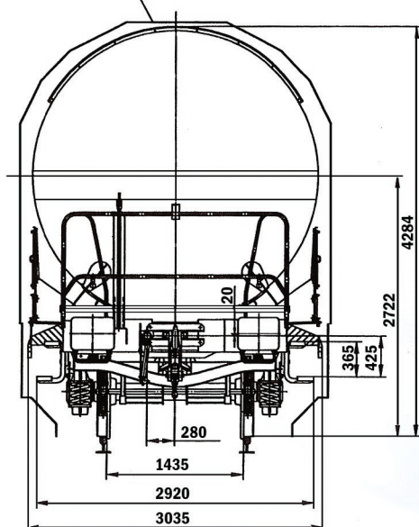
Gabarit UIC 505-1
