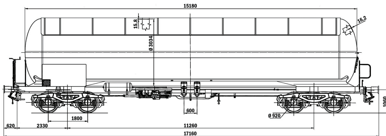
Gabarit UIC 505-1
